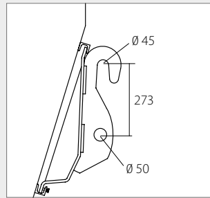
6. Kramer-Allrad Obere Einhängehöhe: 959 mm
