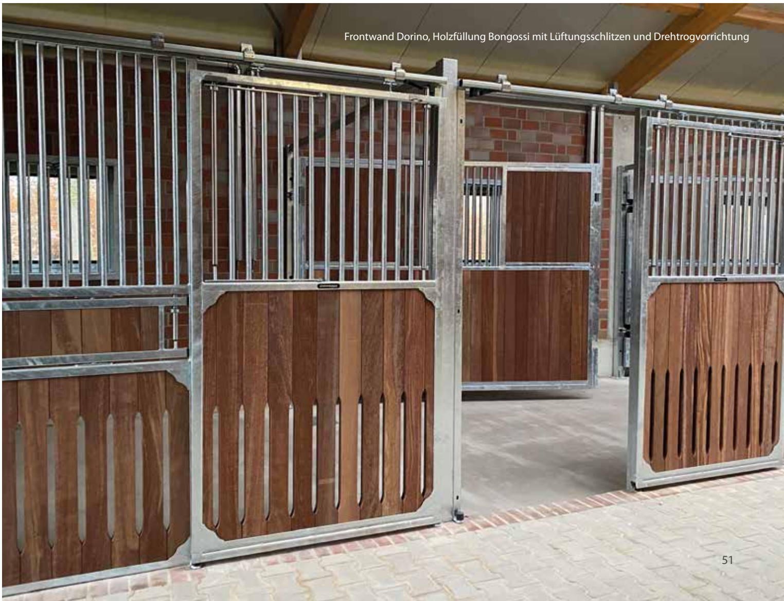
2-teiliges Growi® Stalltor, Vollholz mit Kugelgriff, Holzfüllung Denya 4-teiliges Growi® Stalltor mit Fenster, waagrecht geteilt, mit Drücker, Holzfüllung Denya
