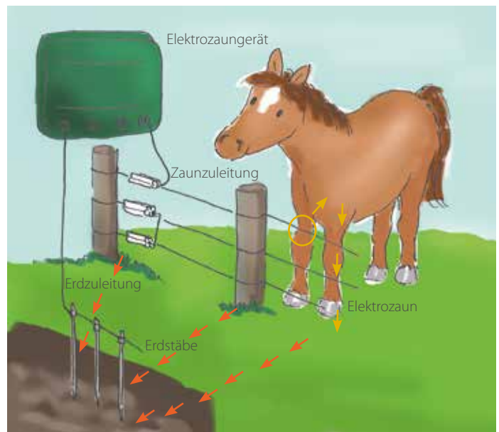
Anwendungsskizze für die Erdung eines Elektrozaungerätes.
