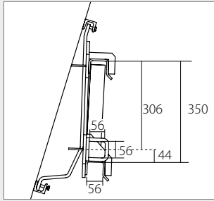
5. Schäffer-Hoflader mechanische Verriegelung Obere Einhängehöhe: 966 mm
